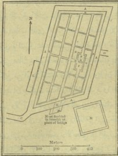
الشكل ١٧٦ الرسم الهندسي الارضي لقرية في شمال ايطاليا قائمة على عُمد
