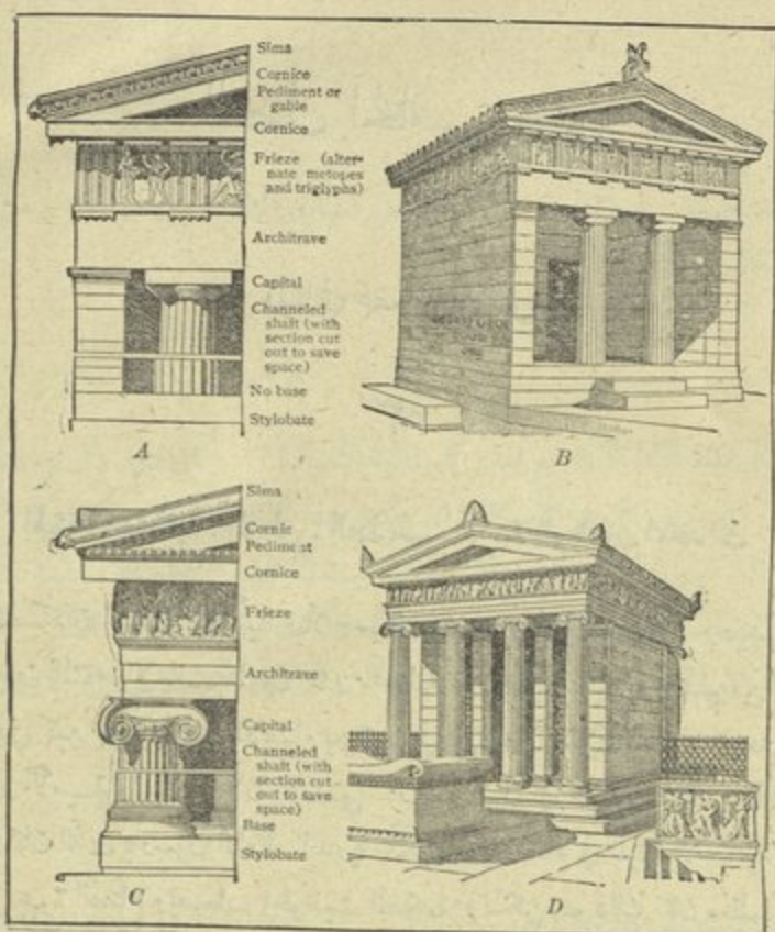
الشكل ١٢٧ يرى هنا رسم الطرازين اليونانيين المهمين في هندسة البناء الطراز الدوري (A و B) والايوني (C و D)
