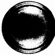
انعراج الأشعة السينية من خلال بلورة .
