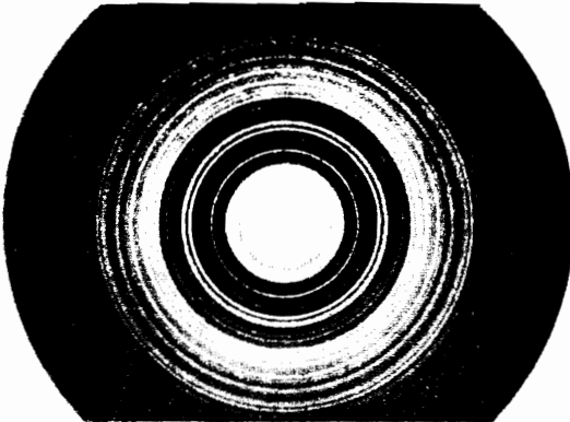
انعراج وابل الكترونات من خلال بلورة .
