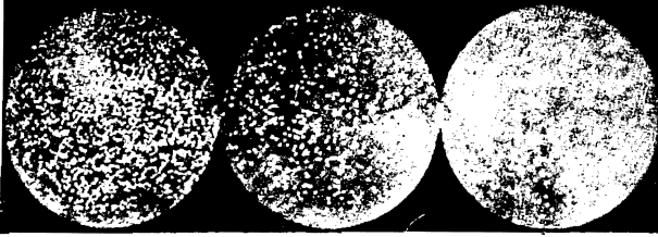
جسيمات براونية كما ترى في المجهر
